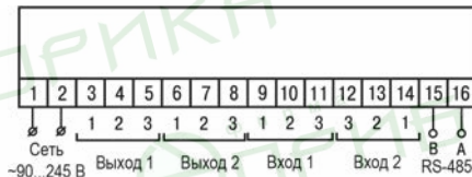
Рисунок 5.2 – Назначение контактов клеммника TRM202-H, -Щ1 и -Щ2
