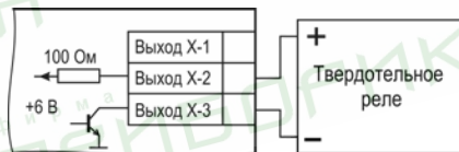
Рисунок 5.14 – Схема подключения нагрузки к ВУ типа Т
