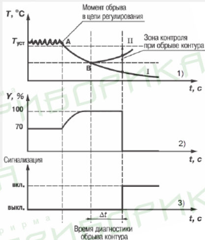
Рисунок 7.11 – Срабатывание LBA
