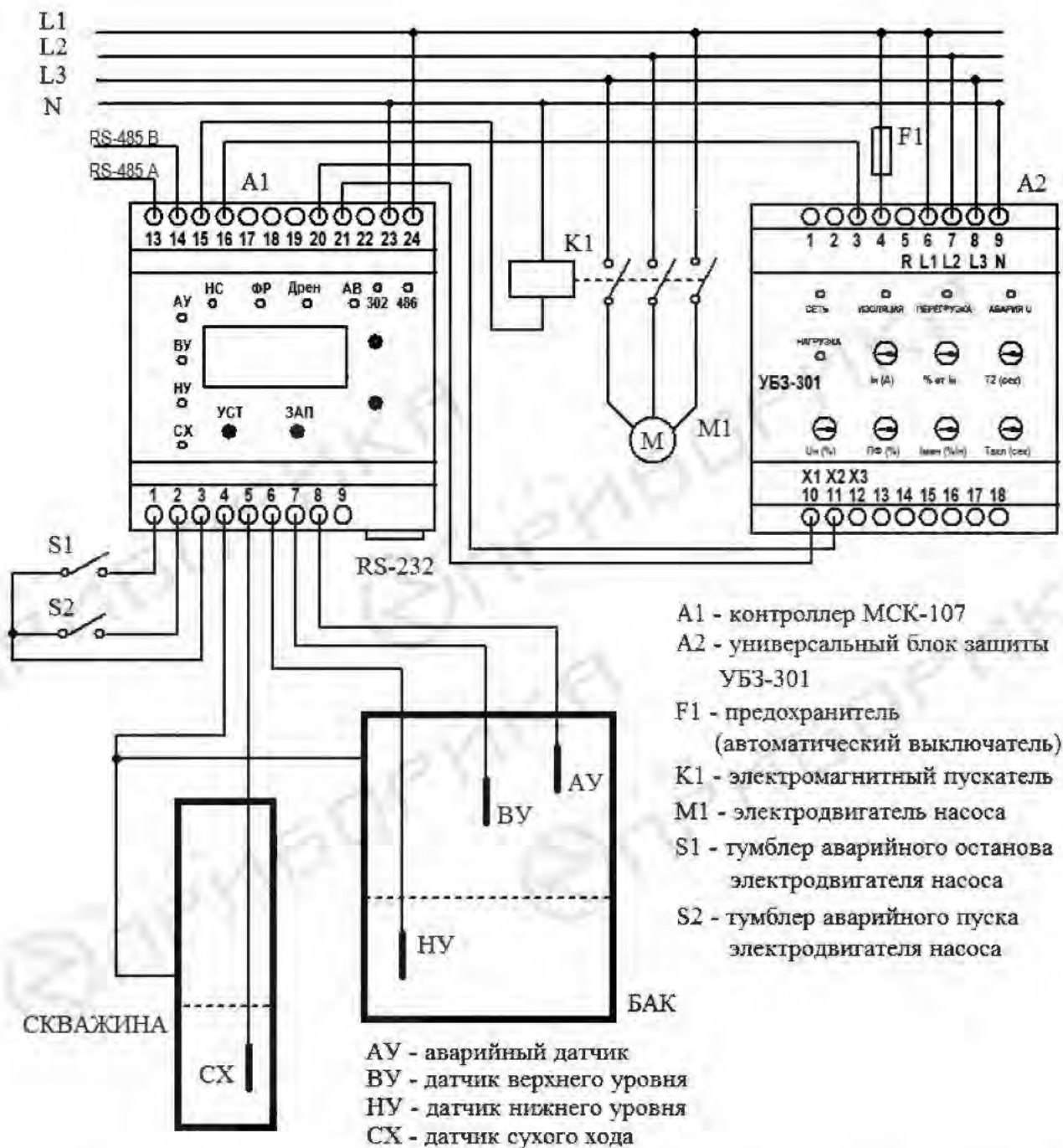
Рисунок 2 – Схема подключения MCK-107 при использовании кондуктометрических датчиков
