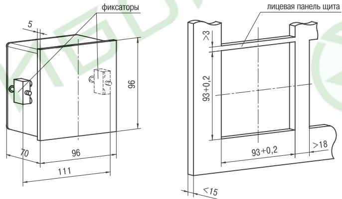
Рис. А.2. Корпус щитового крепления типа ЩЦ1
