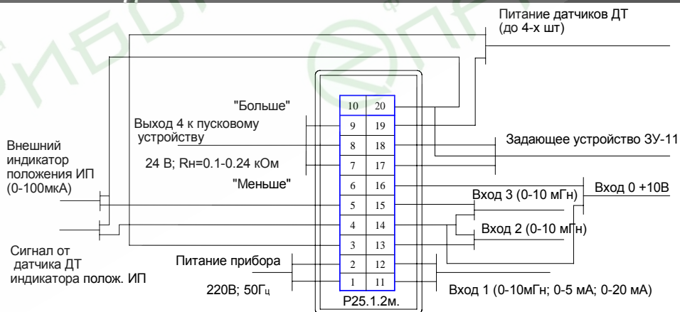
Схема подключения прибора Р25.1.2м.
